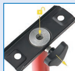
Schnellverschluss zur Aufnahme des Doppelträgers
